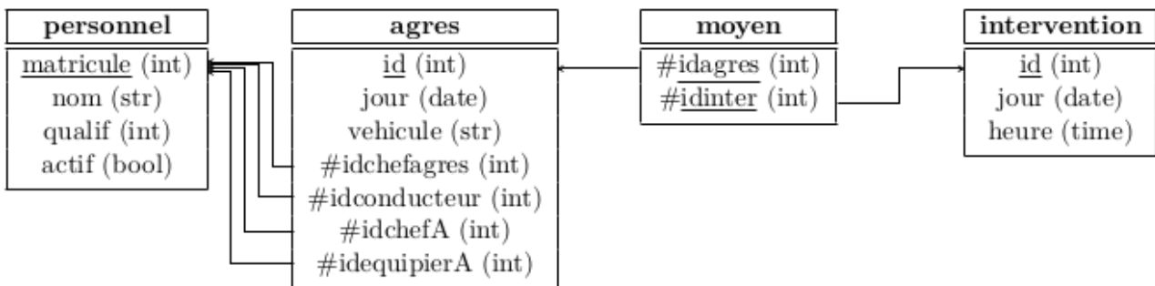
Figure 1. Schéma relationnel
