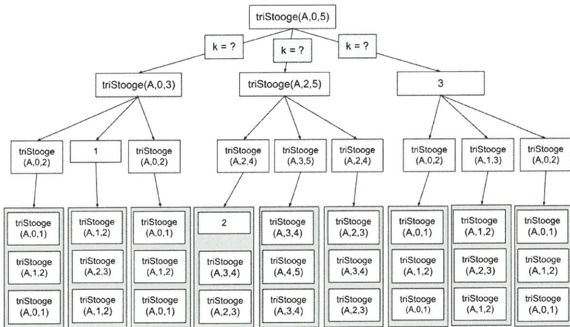
Figure 1. Arbre des appels récursifs pour \text{triStooge}(A, 0, 5)
